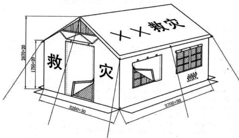
图1 样式、结构及主要尺寸
