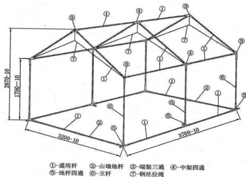
图2 框架各部件名称、结构及主要尺寸
