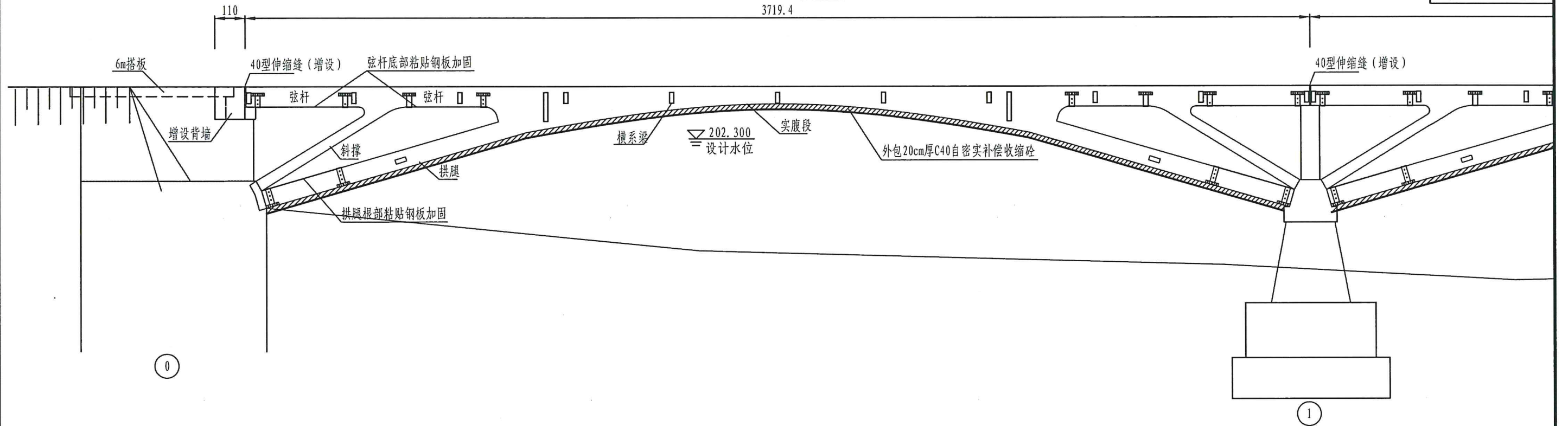
立面 1:150
