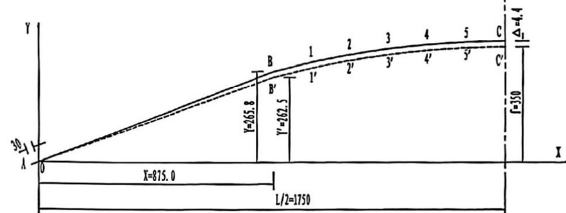
拱片内缘坐标设置示意图
