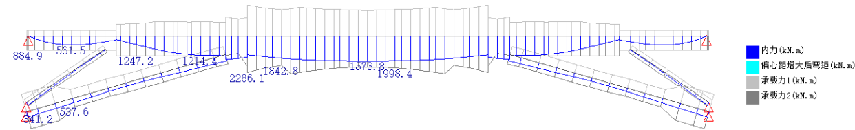
图 8 加固后承载能力极限状态最大弯矩分布
