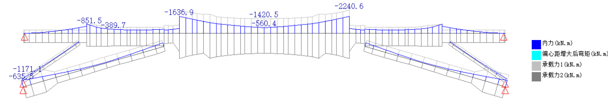
图 9 加固后承载能力极限状态最小弯矩分布
