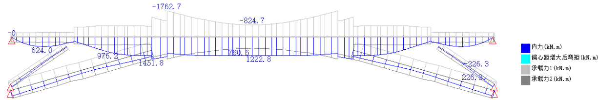
图 5 现行规范承载能力极限状态最大弯矩分布
