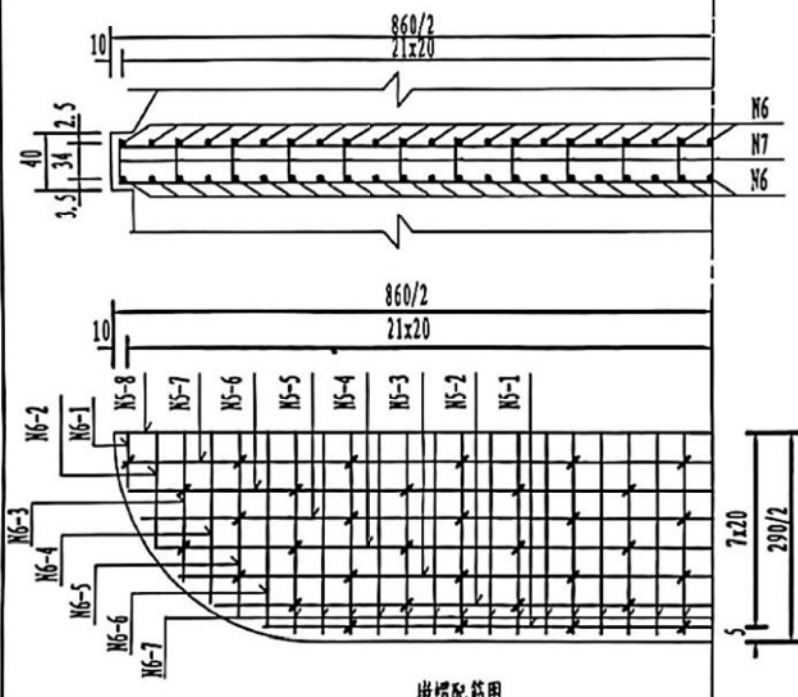
墩帽配筋图
