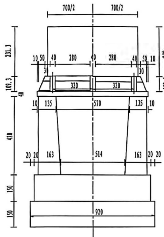
半正面 (西侧)
