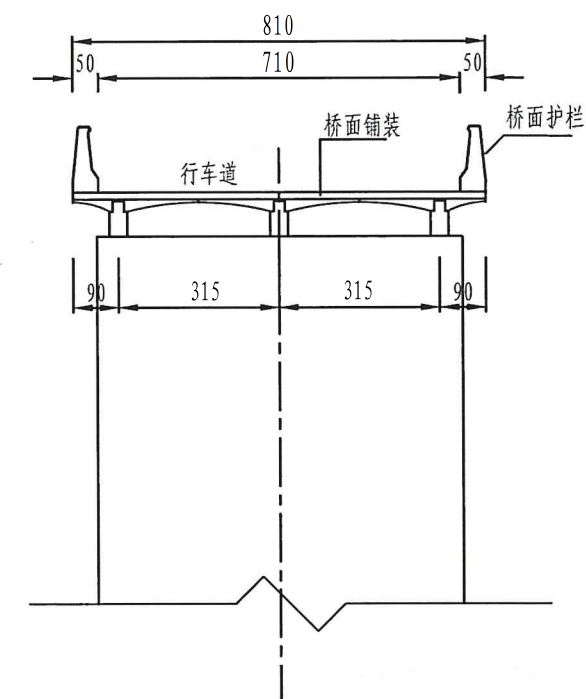
断面 1:150
