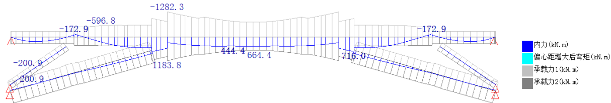
图 4 1985 规范承载能力极限状态最大弯矩分布
