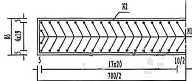
桥墩配筋图
