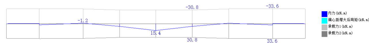
图 13 跨中横隔梁最大正弯矩分布图
