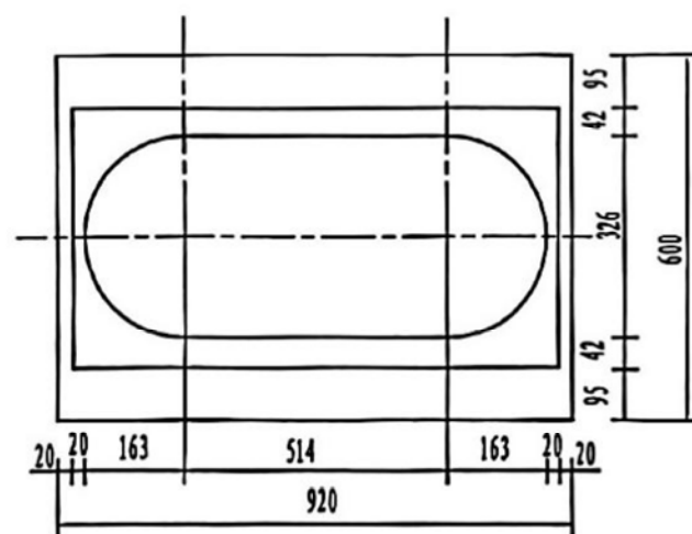
基顶平面
