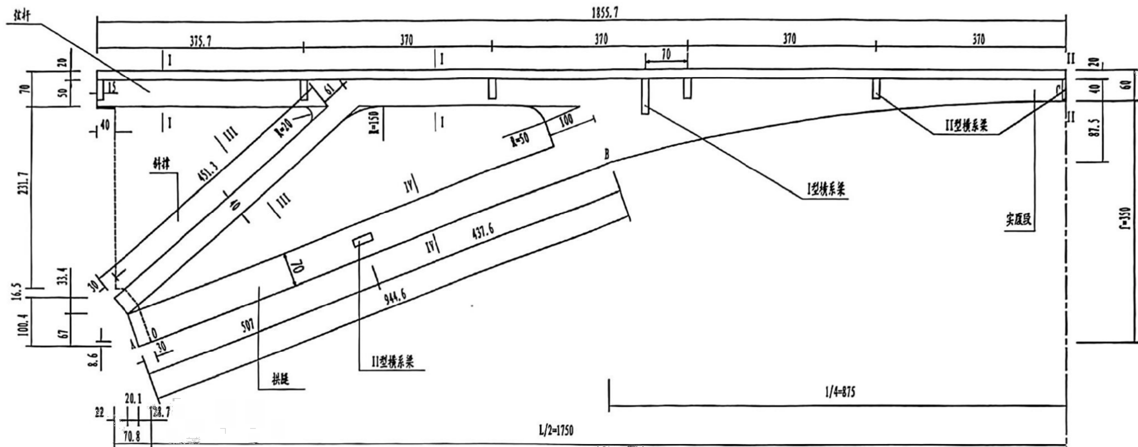
拱片半立面图
