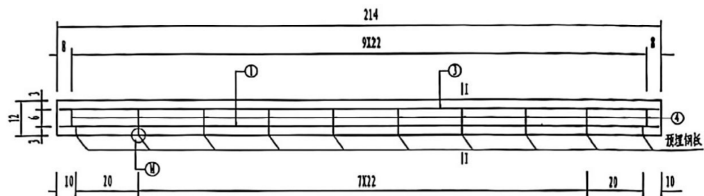
扶手
