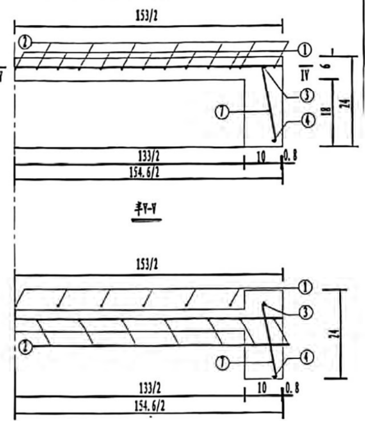
半V-V
