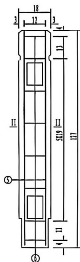
中栏杆柱
