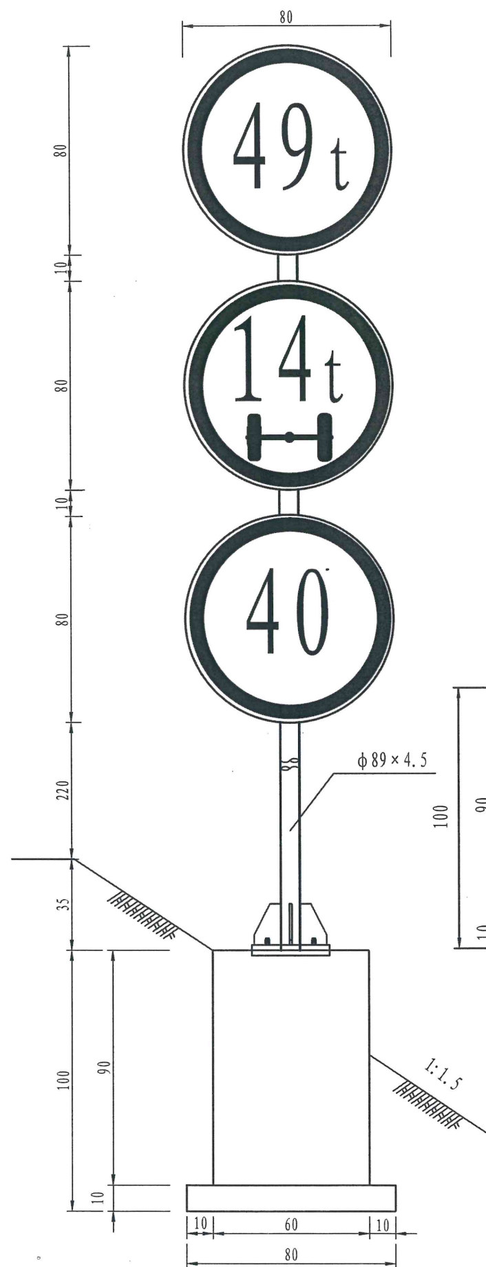
标志立面图 (1:20)
