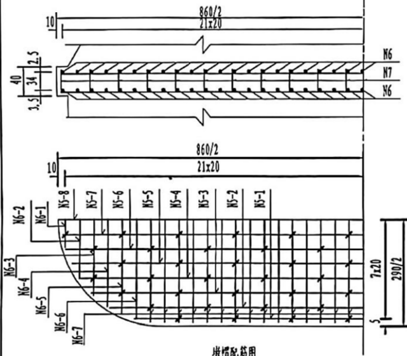
墩帽配筋图
