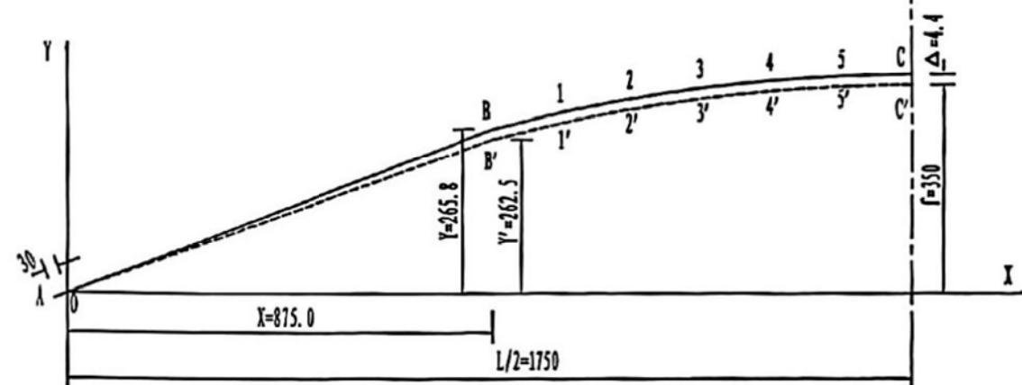
拱片内缘坐标尺寸示意图
