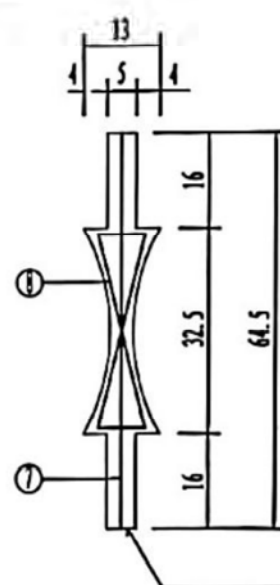
中栏杆
