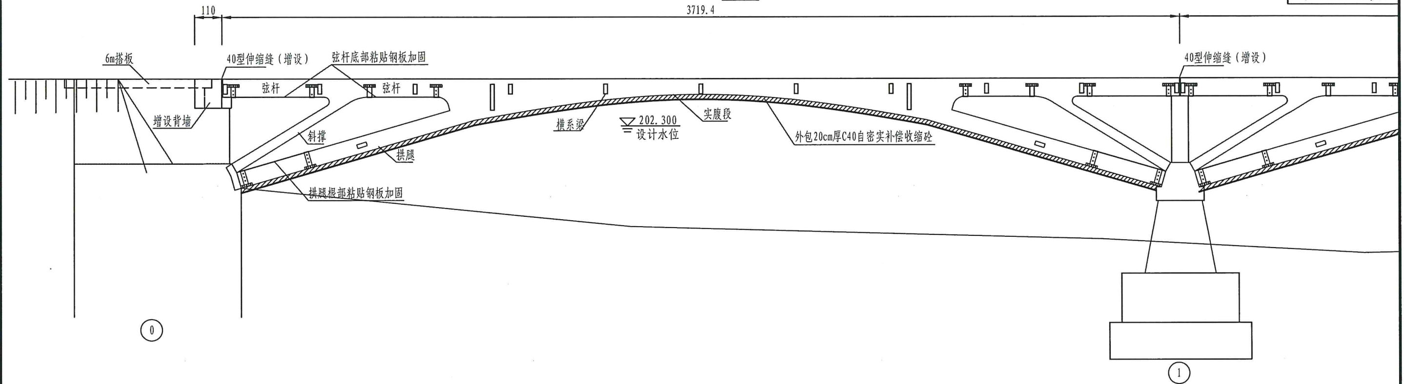
立面 1:150
