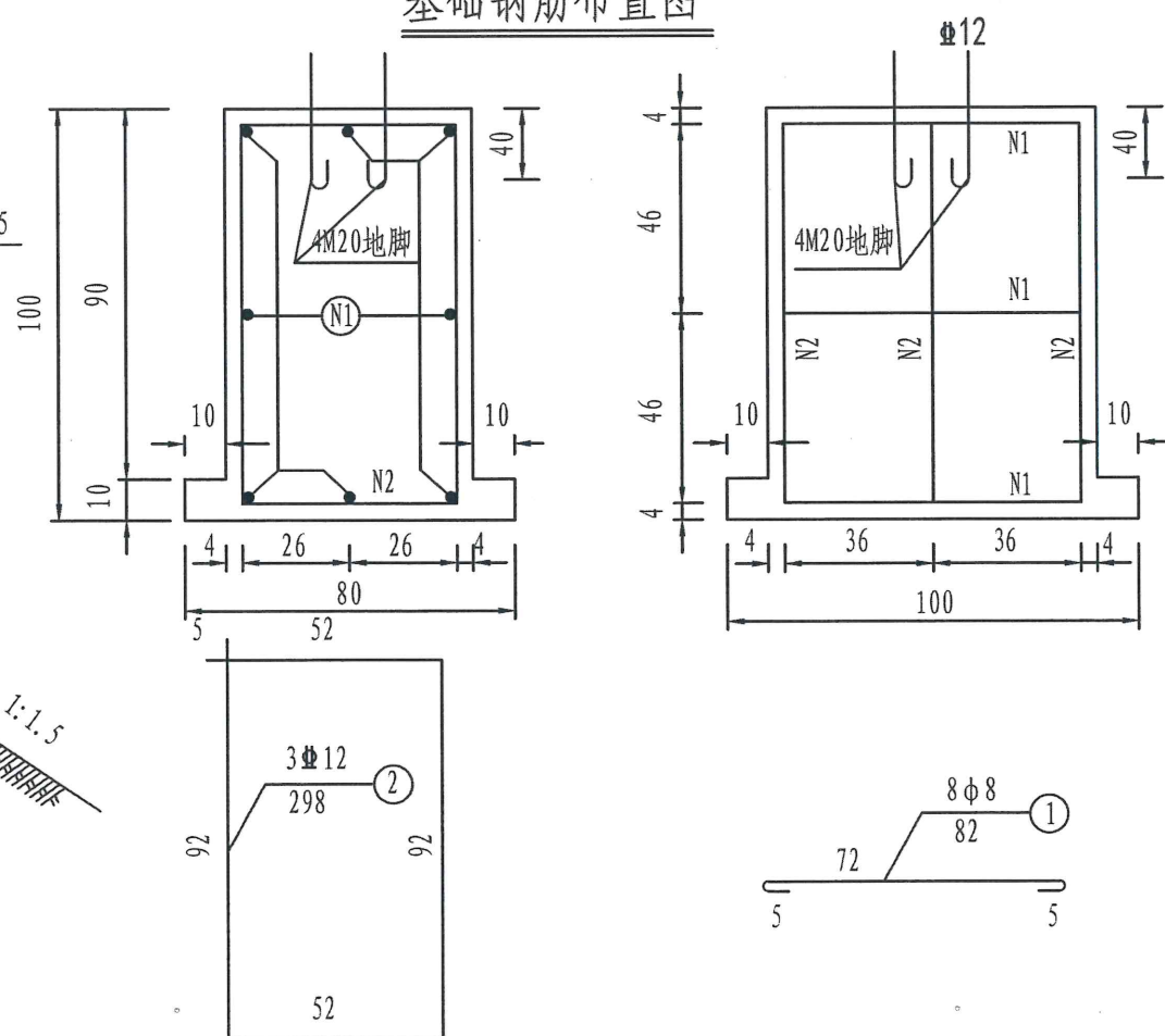
基础钢筋布置图
