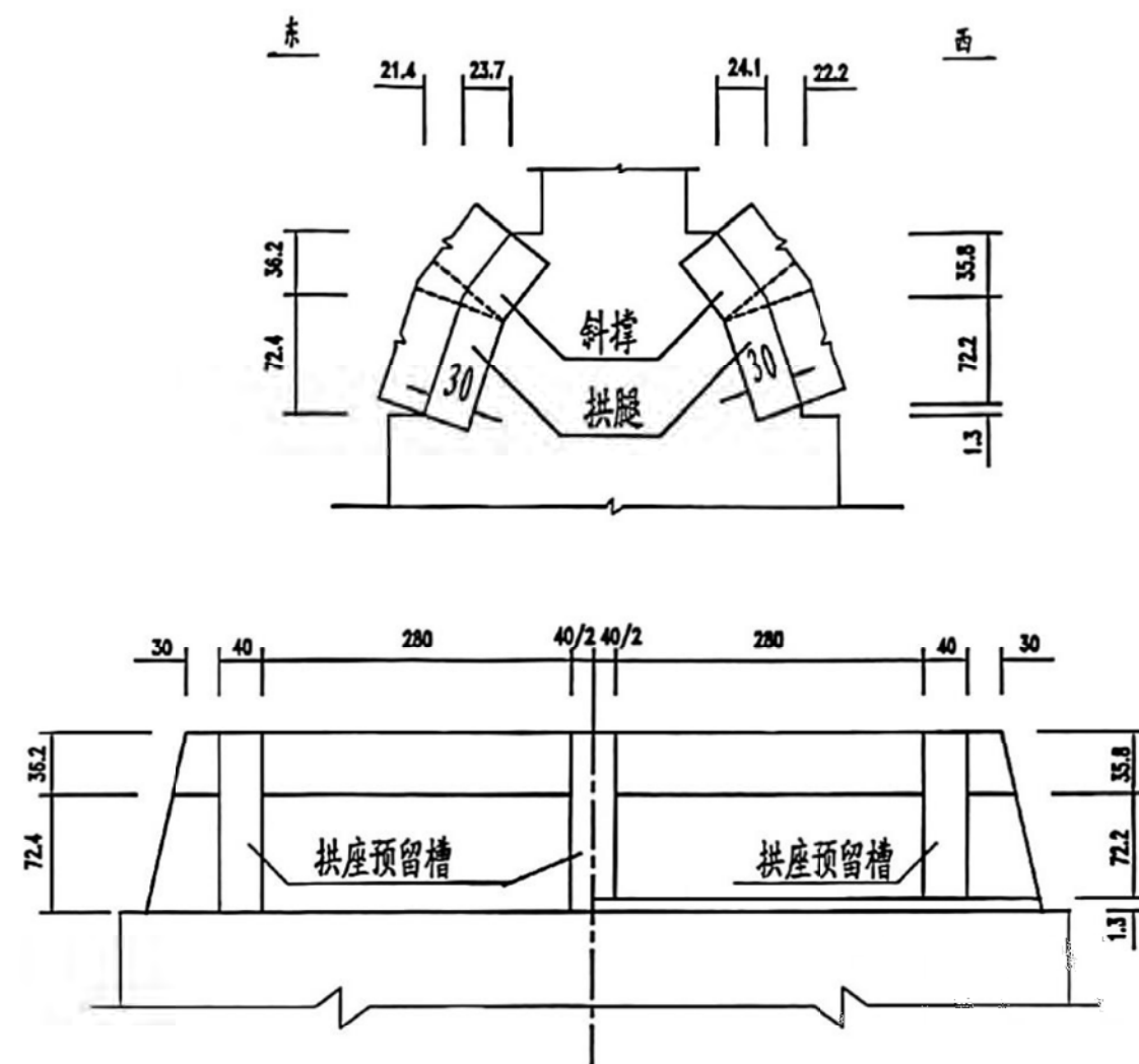
拱座大样
