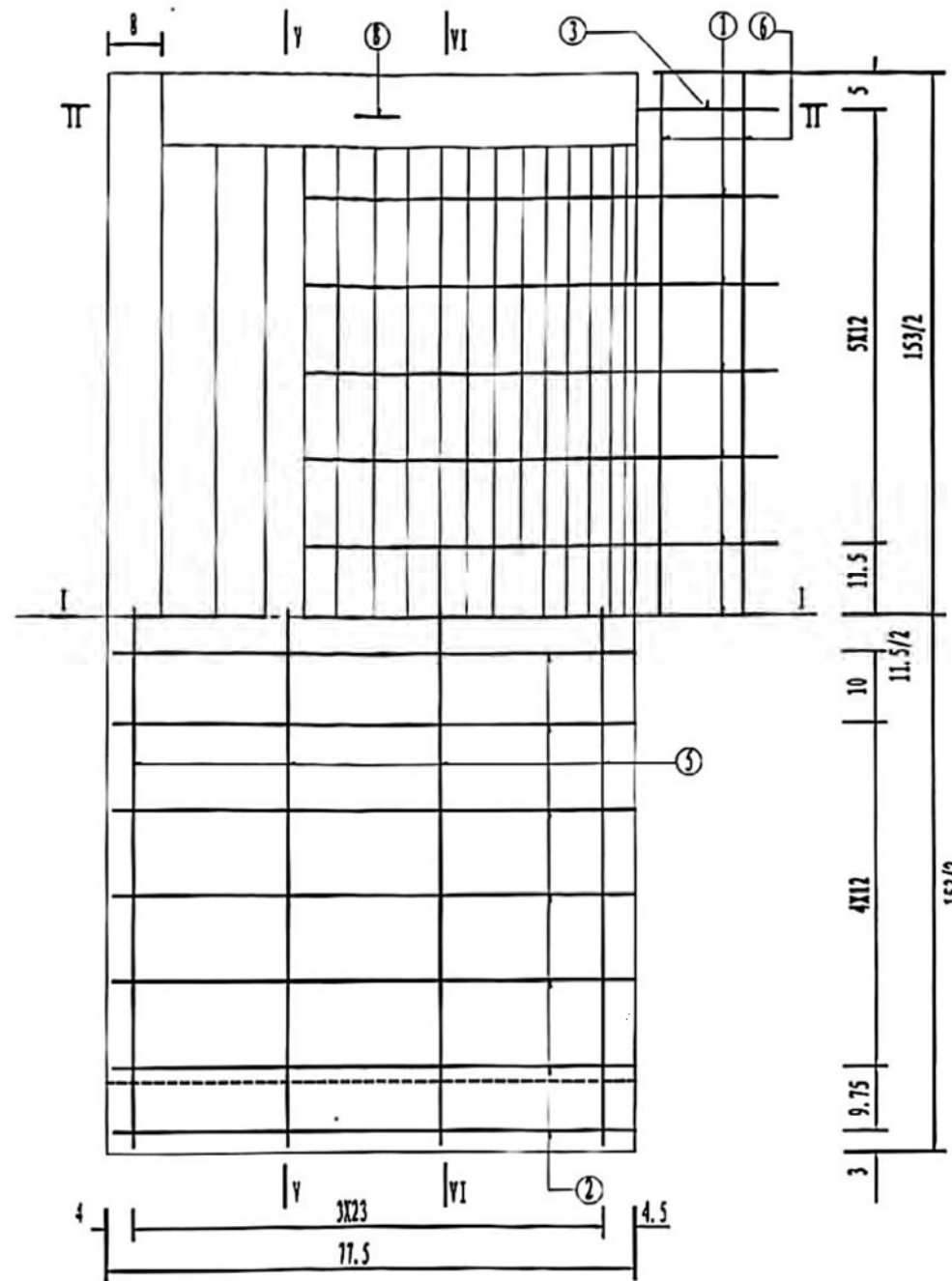
半III-III
