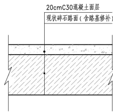
机动车道路面结构
